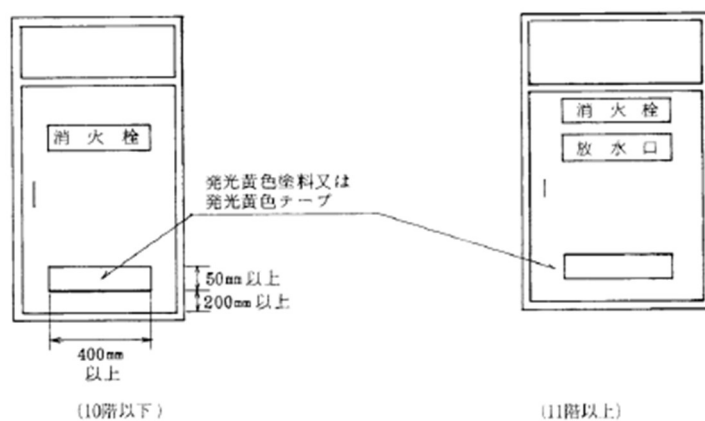
③ 屋内消火栓，連結送水管放水口併用型
